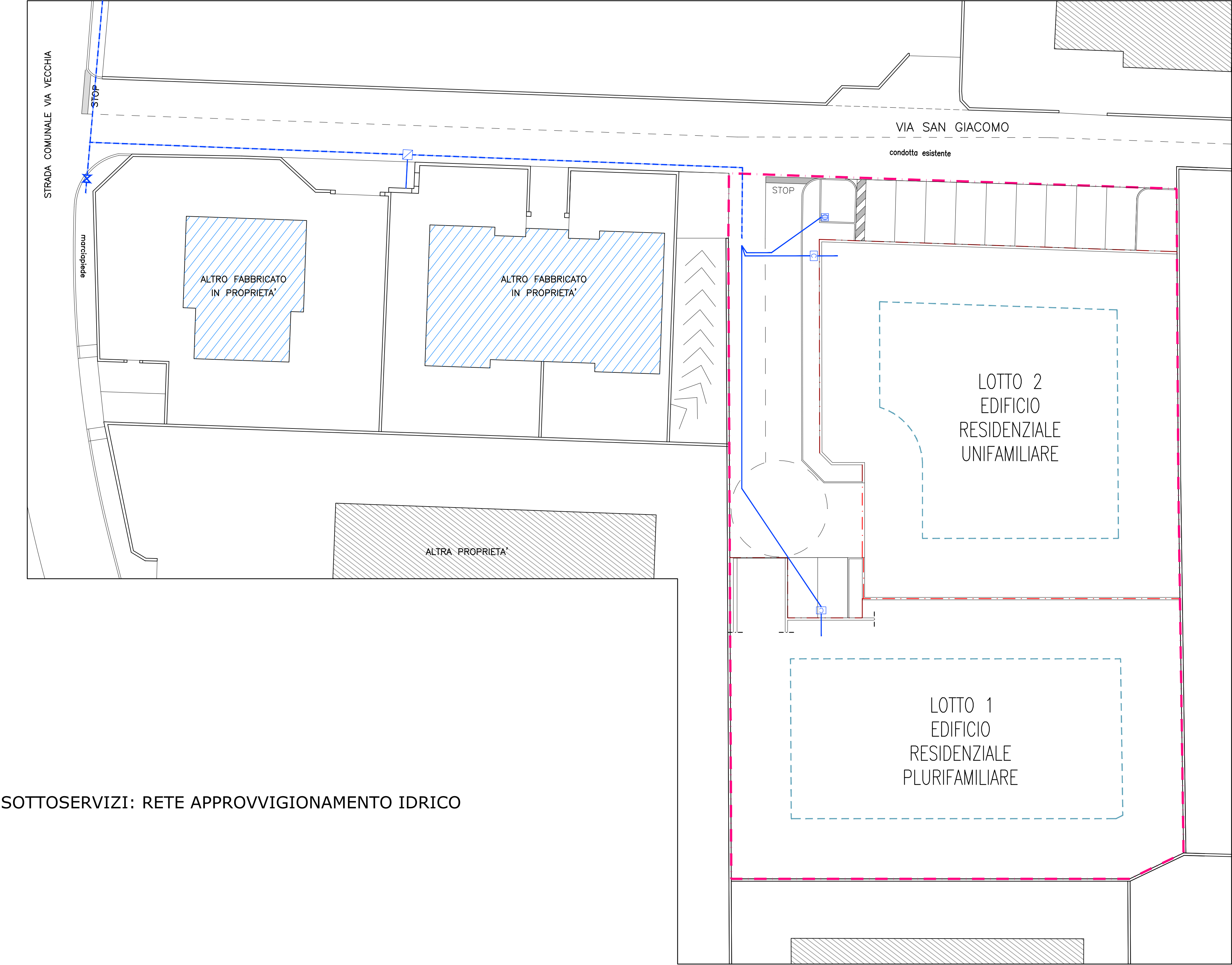
PLANIMETRIA DI PROGETTO APPROVVIGIONAMENTO IDRICO scala 1:200
